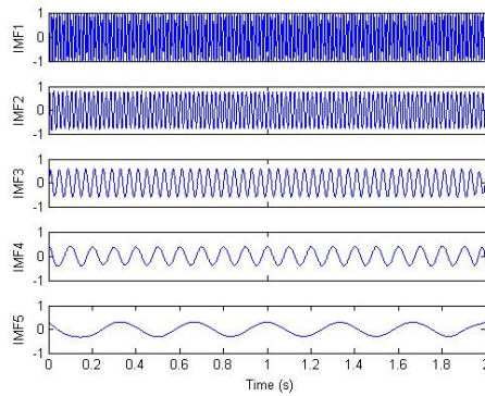
(b) IMFs
